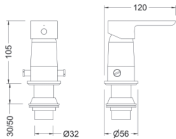
Ref.: 65142 19 45 66 Monomando de bidé con transmisión Single lever bidet mixer with diverter
