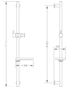
Ref.: 1639 45 Barra ducha metálica Metallic shower bar
