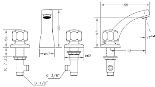
Ref.: 68120 11 45 66 Batería de lavabo Widespread wash-basin mixer
