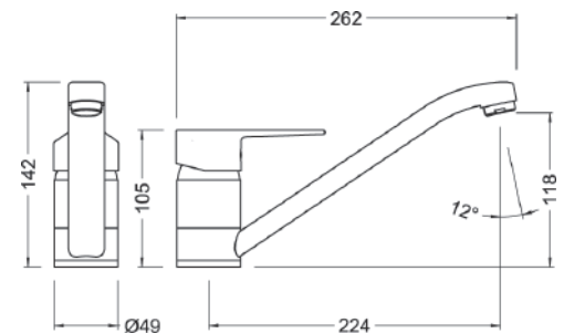
Ref.: 61200 28 45 66 Monomando de fregadera Single lever sink mixer
