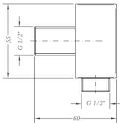
Ref.: 1679 04 Toma ducha mural cuadrada Square wall flexible connector Box: 1 | Carton: 96 | Pallet: 2304
