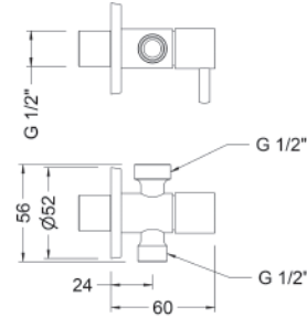
Ref.: 3107 04 Válvula de escuadra doble 1/2" - 1/2" ducha- inodoro Double angle valve 1/2" - 1/2" Box: 1 | Carton: 160 | Pallet: 3840
