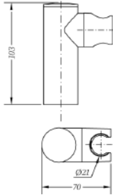
Ref.: 100153 45 Soporte ducha cilíndrico Cylindrical shower holder
