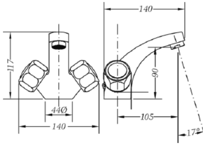
Ref.: 68130 11 45 66 Monobloc de lavabo Wash-basin mixer
