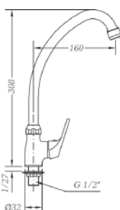
Ref.: 1009 04 Grifo fregadera 1 agua cartucho 25 One-water sink tap 25 cartridge
