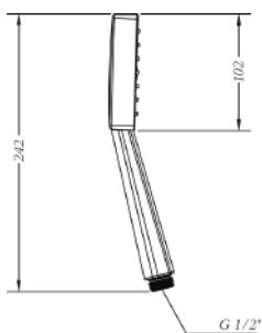
Ref.: DXK1 45 Mango de ducha K1 jets K1 jet handshower
