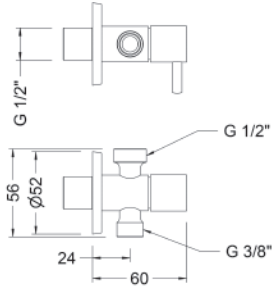
Ref.: 3107 03 Válvula de escuadra doble 1/2" - 3/8" ducha- inodoro Double angle valve 1/2" - 3/8" Box: 1 | Carton: 160 | Pallet: 3840
