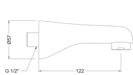
Ref.: 1667 45 Caño mural baño fundido Casted wall bath spout Box: 1 | Carton: 60 | Pallet: 1080
