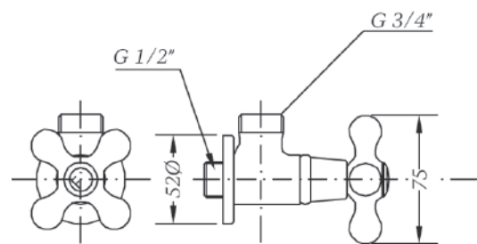
Ref.: 568575 45 Cuerpo grifo mural Wall body tap
