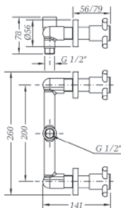
Ref.: 68115 08 45 66 Grupo ducha empotrado 8" Built-in 8" shower mixer
