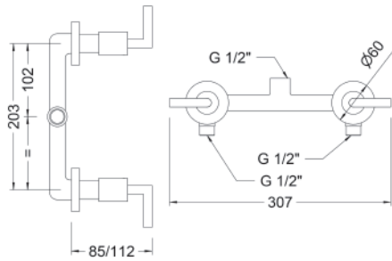
Ref.: 68115 12 45 66 Grupo ducha empotrado 8\"/> Built-in 8" shower mixer
