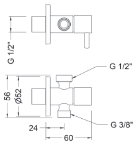
Ref.: 3108 03 Válvula de escuadra doble 1/2" - 3/8" Inox SS double angle valve 1/2" - 3/8" Box: 1 | Carton: 160 | Pallet: 3840
