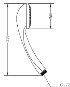
Ref.: 100175 45 00 Mango de ducha E1 jet E1 jet handshower
