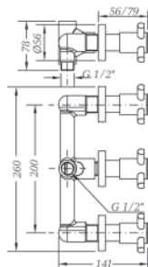
Ref.: 68116 08 45 66 Grupo ducha empotrado 8" con inversor Built-in 8" bath mixer with diverter
