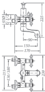
Ref.: 68526 09 43 66 Mezclador de baño bronce con kit Bronze bath mixer with kit
