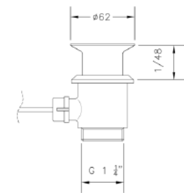
Ref.: 100200 45 Válvula automática plástico 1 1/4" 1 1/4" plastic automatic valve
