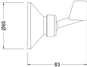
Ref.: 1647 45 Soporte ducha Clásico Classic shower holder
