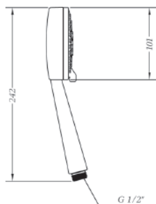
Ref.: DXK3 45 Mango de ducha K3 jets K3 jets handshower
