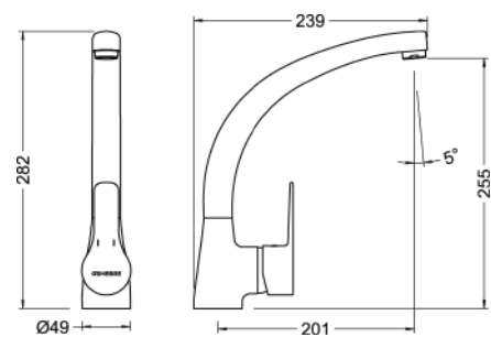
Ref.: 61201 28 45 66 Monomando de fregadera caño fundido Single lever sink mixer casted spout
