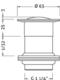
Ref.: 100207 45 Válvula click 1 1/4" 1 1/4" click valve
