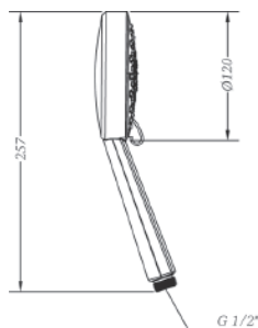
Ref.: DXT5 45 Mango de ducha T5 jets T5 jets handshower
