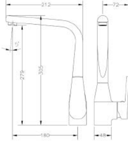
Ref.: 64201 16 45 66 Monomando de fregadera Single lever sink mixer
