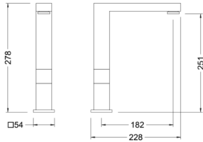
Ref.: 65208 18 60 66 Monomando de fregadera inox con cartucho progresivo Stainless steel sink mixer with progressive cartridge
