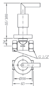
Ref.: 68170 12 45 66 Llave de paso 1/2\"/> Stopcock 1/2"
