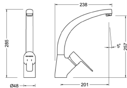
Ref.: 61204 28 45 66 Monomando de fregadera caño conformado Single-lever sink mixer tube spout
