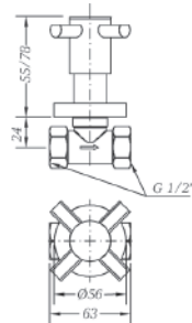
Ref.: 68170 08 45 66 Llave de paso 1/2" Stopcock 1/2"
