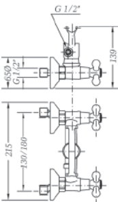
Ref.: 68531 09 45 66 Mezclador de ducha cromo con kit Chromed shower mixer with kit
