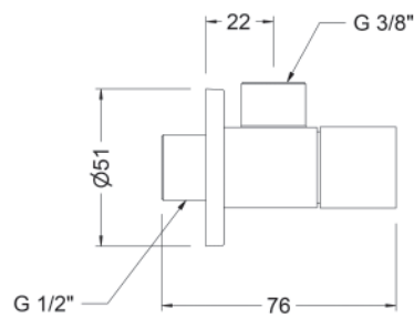
Ref.: 3106 05 Válvula de escuadra cuadrada 1/2" Square angle valve 1/2" Box: 2 | Carton: 120 | Pallet: 4320
