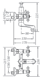
Ref.: 68526 09 45 66 Mezclador de baño cromo con kit Chromed bath mixer with kit
