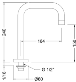
Ref.: 68915 45 Caño encimera recto tubo Straight pipe spout
