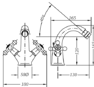
Ref.: 68516 09 45 66 Monobloc de bidé cromo Chromed bidet mixer
