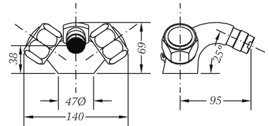
Ref.: 68140 11 45 66 Monobloc de bidé Bidet mixer
