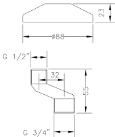
Ref.: 100122 45 Conjunto florón y excéntricas gigantes Giant escutcheon eccentric set
