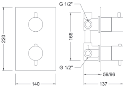
Ref.: 64111 14 45 67 Termostática empotrada 3 vías Built-in 3-way thermostatic
