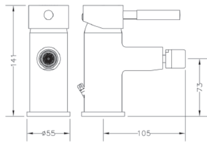
Ref.: 65145 18 45 66 Monomando de bidé Single lever bidet mixer
