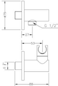
Ref.: 1633 04 Soporte ducha con toma cilíndrico Round flexible wall conector
