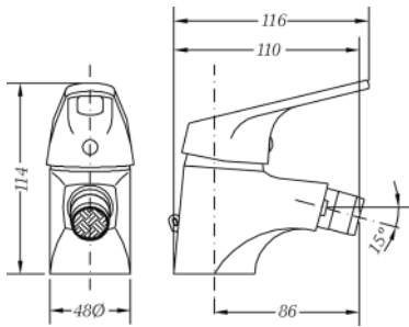
Ref.: 60140 22 45 66 Monomando de bidé Single lever bidet mixer
